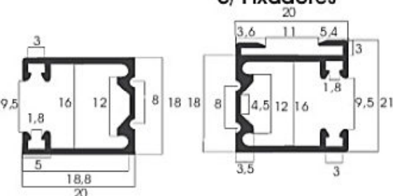
Guia Lateral Fixação Directa Fixação Frontal c/ Fixadores
